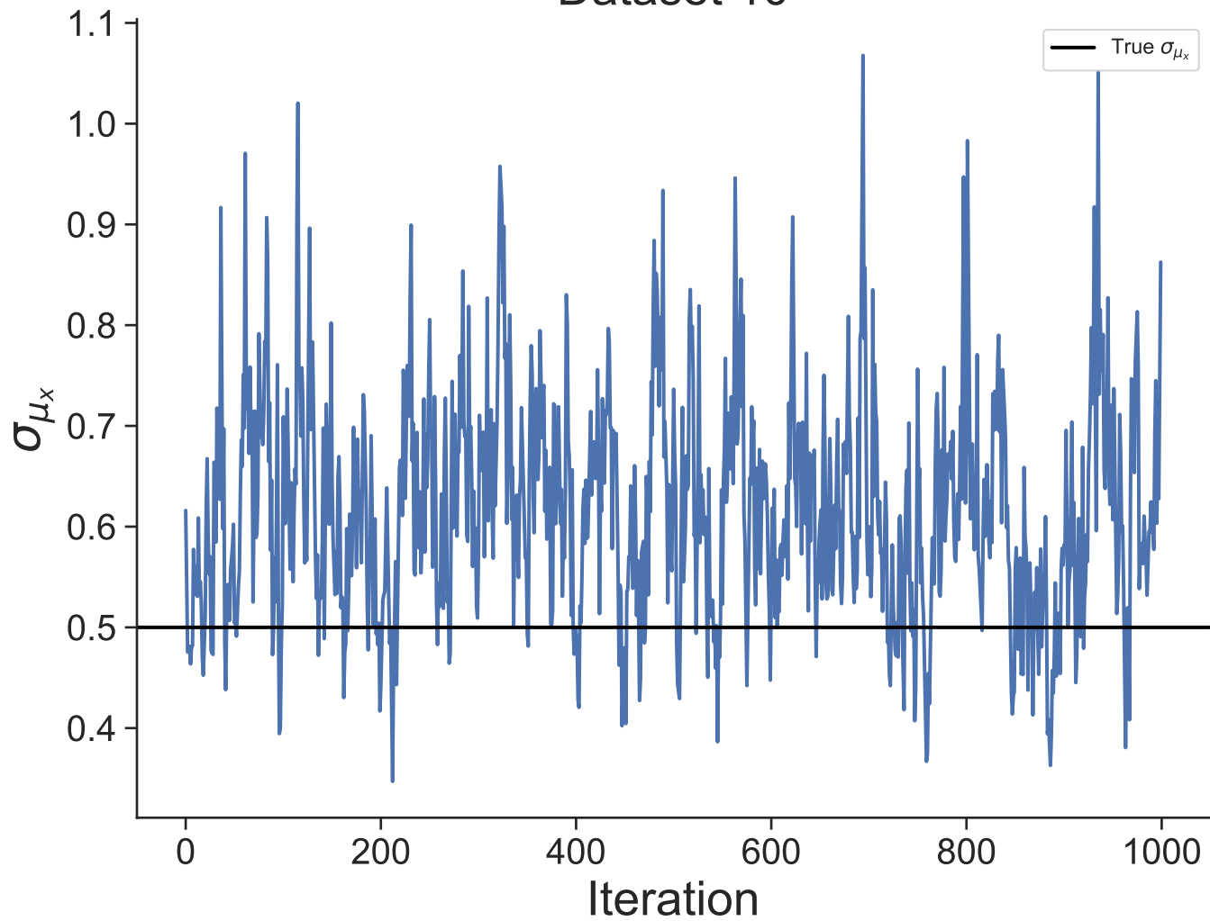
Dataset 10
