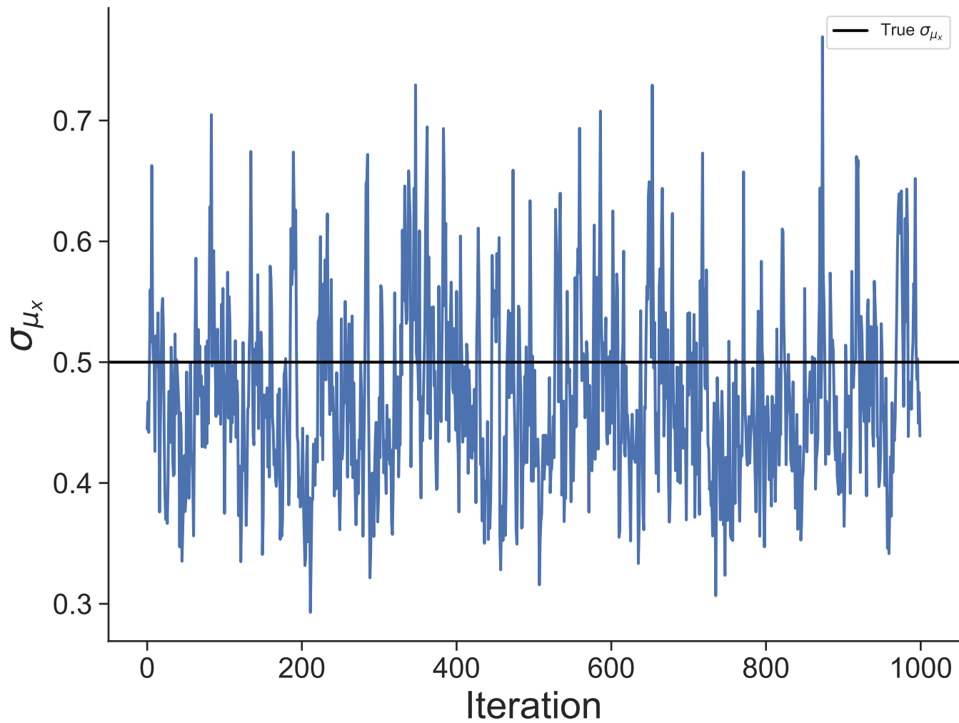
Dataset 11
