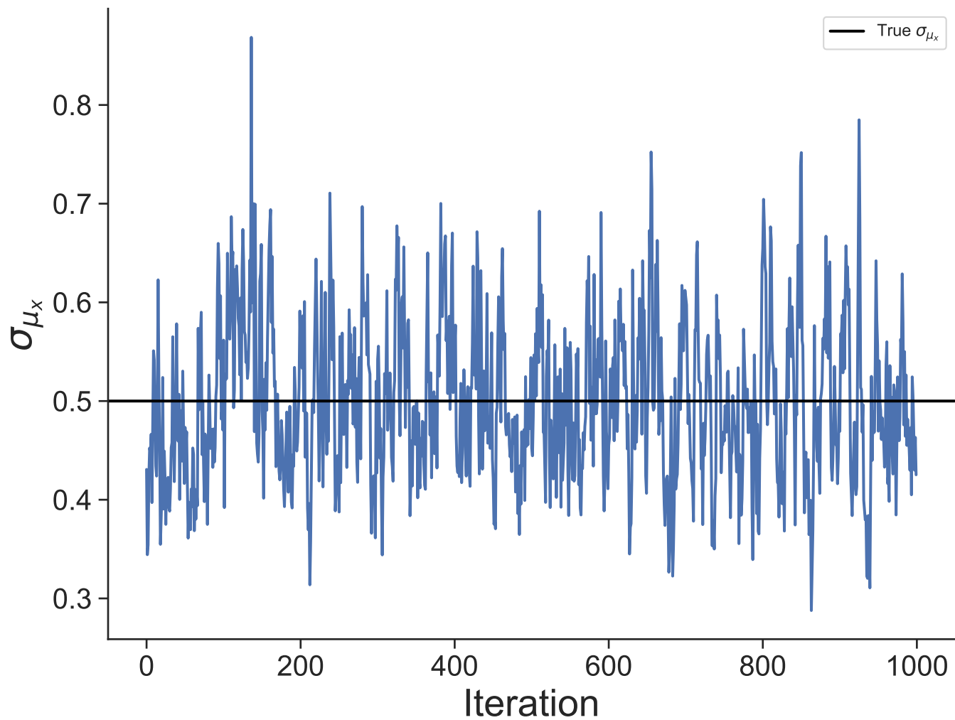
Dataset 48
