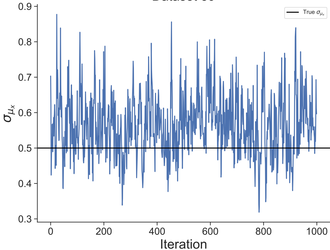
Dataset 39
