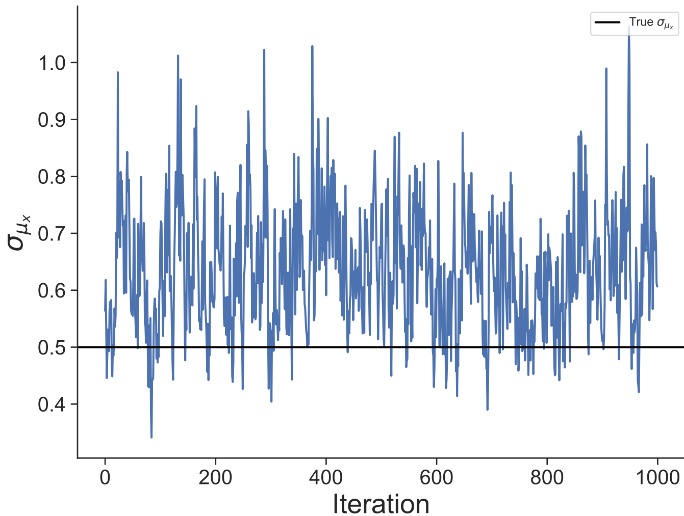
Dataset 22
