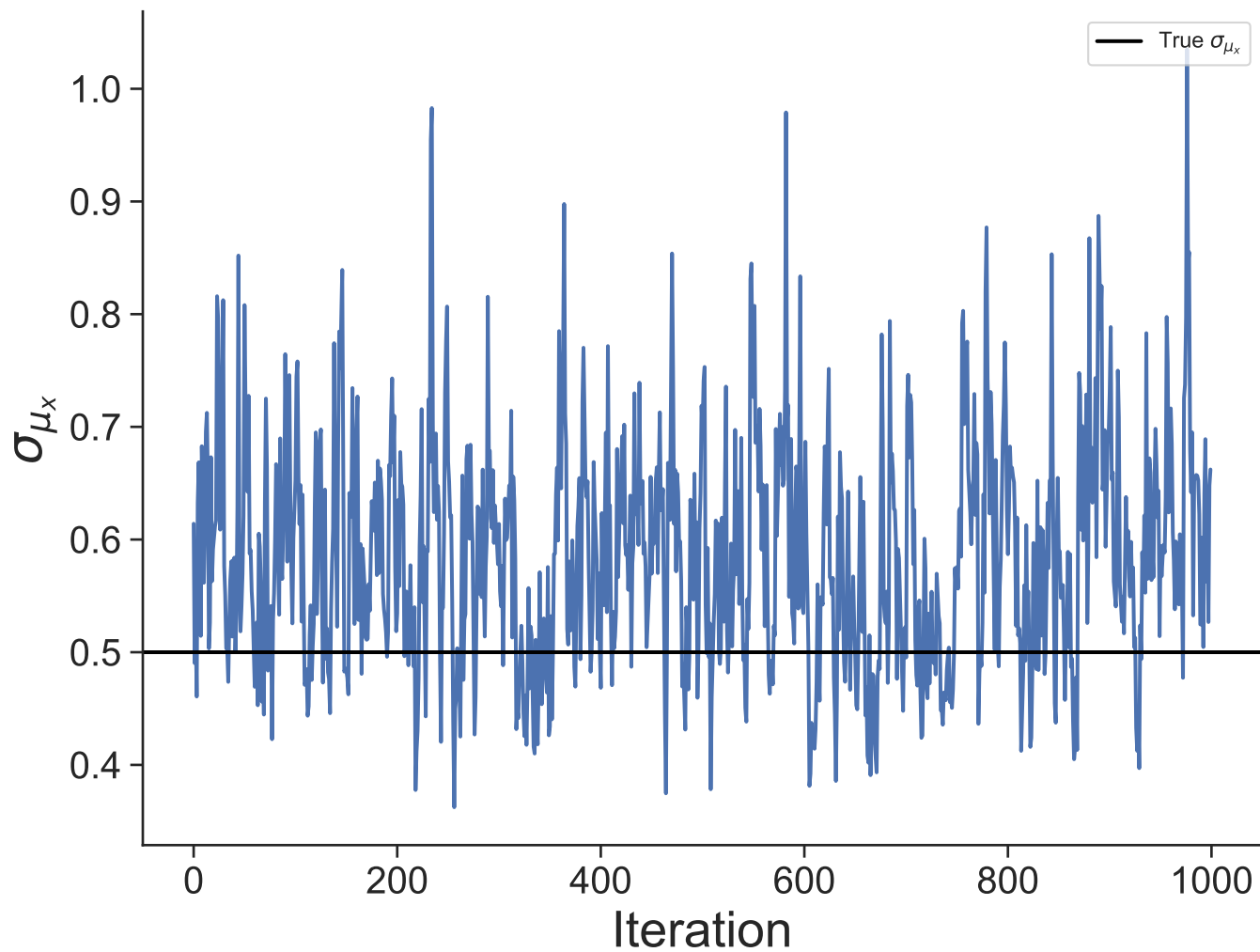
Dataset 46
